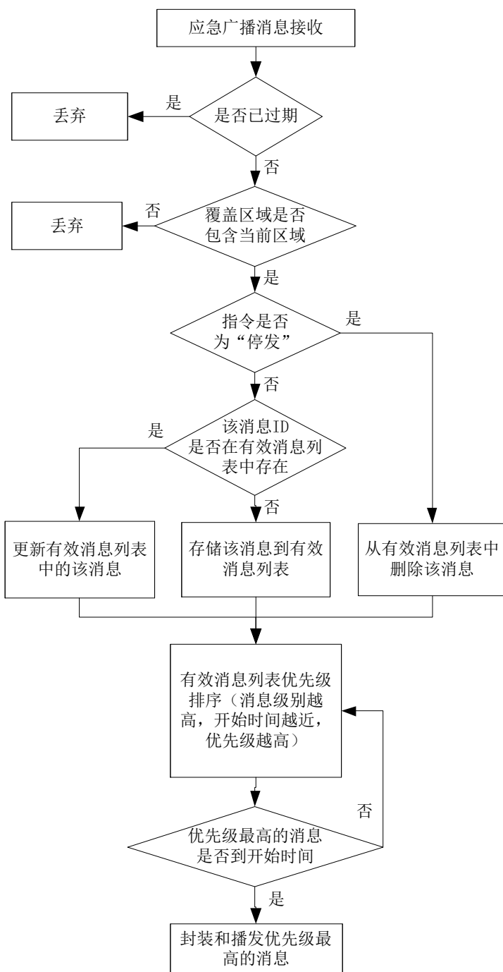
图 B.1 应急广播适配器对应急广播消息的处理流程示例
