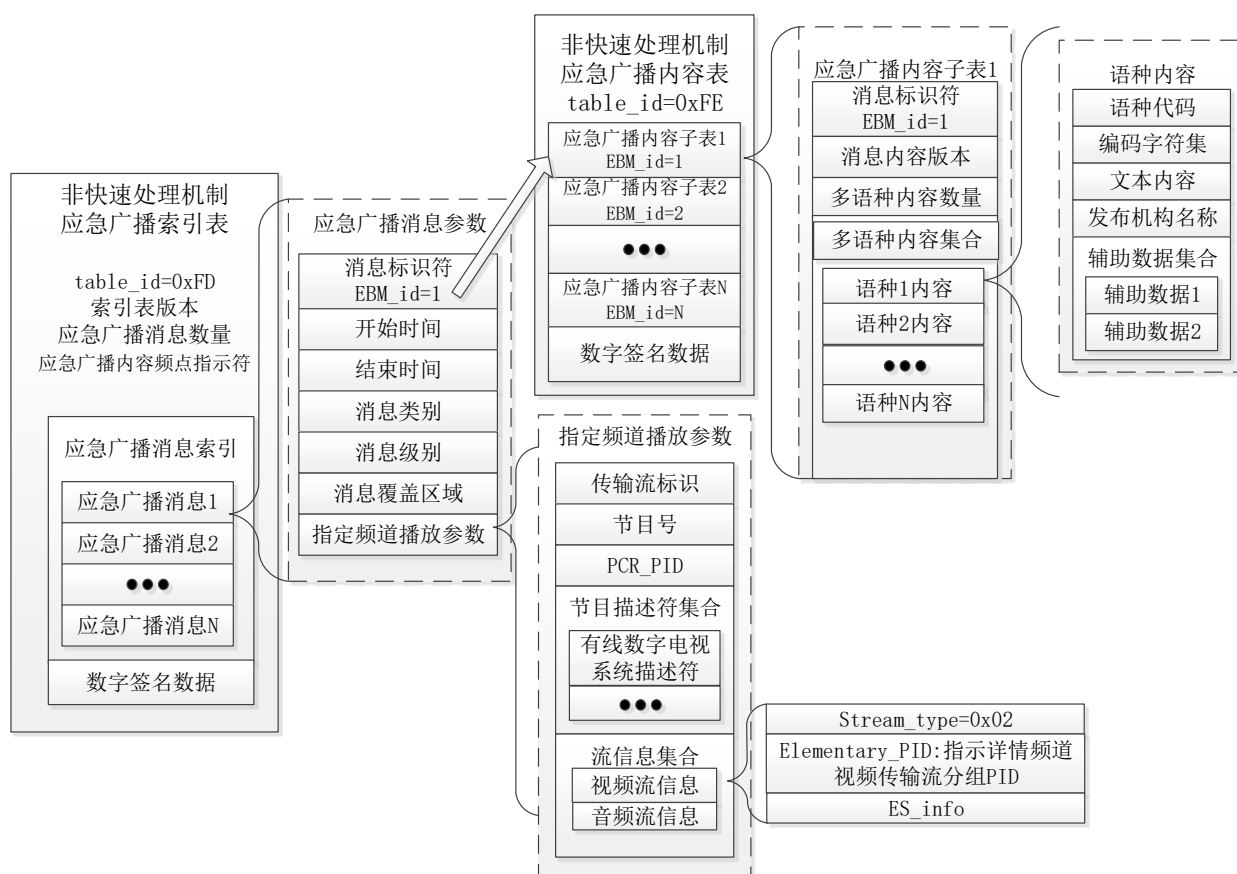
图2 非快速处理机制应急广播索引表和非快速处理机制应急广播内容表的关系
