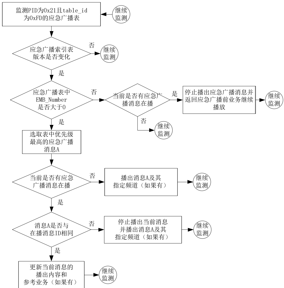
图 B.2 终端对应急广播消息的处理流程示例
