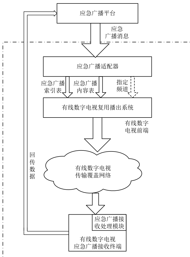
图1 有线数字电视应急广播系统架构
